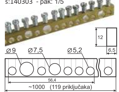
Stezaljka 119 x 16/25/35 100A š:140303 - pak: 1/5
