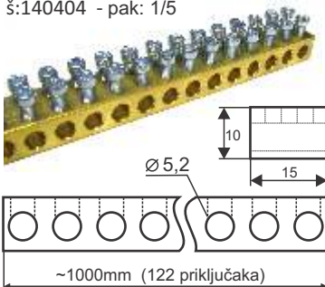
Stezaljka 122 x 16mm 200A š:140404 - pak: 1/5
