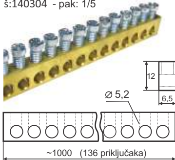
Stezaljka 136 x 16mm 2 100A š:140304 - pak: 1/5
