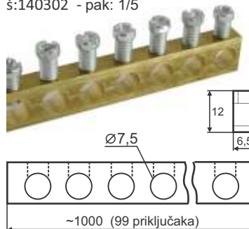
Stezaljka 104 x 25mm 2 100A š:140302 - pak: 1/5
