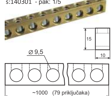
Stezaljka 79 x 35mm 2 200A š:140301 - pak: 1/5
