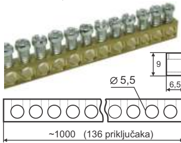
Stezaljka 136 x 16mm 2 63A š:140206 - pak: 1/10
