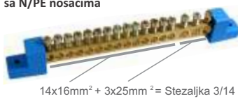
14x16mm 2 + 3x25mm 2 = Stezaljka 3/14 PE
