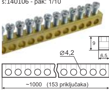
Stezaljka 153 x 10mm 2 63A š:140106 - pak: 1/10
